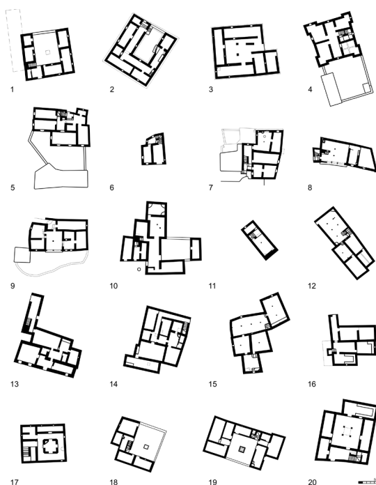
Figura 3. Levantamento. Tipologias da arquitetura doméstica nas montanhas do Atlas em Marrocos
