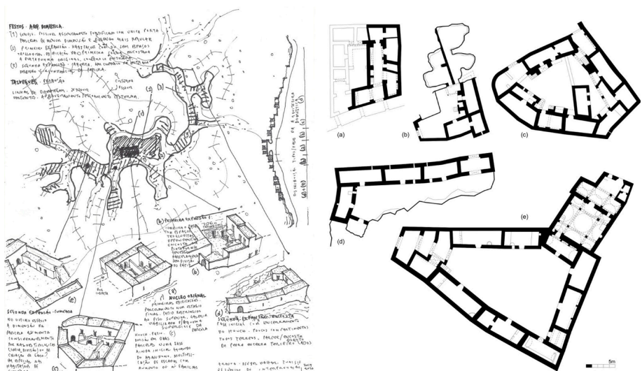
Figura 10. Zraoua: urbanismo e arquitetura
