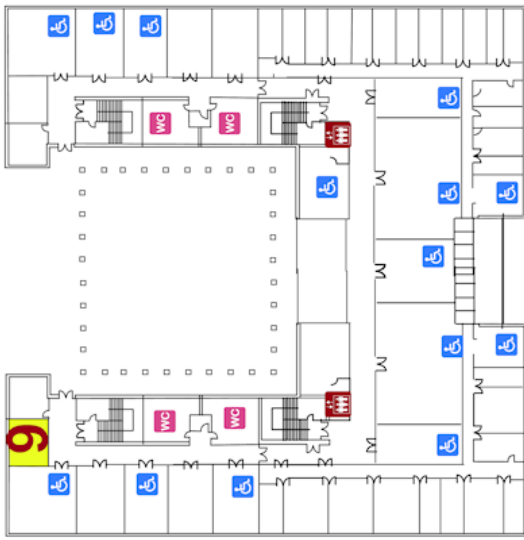
PLANTA 1 1. SOLAIRUA
